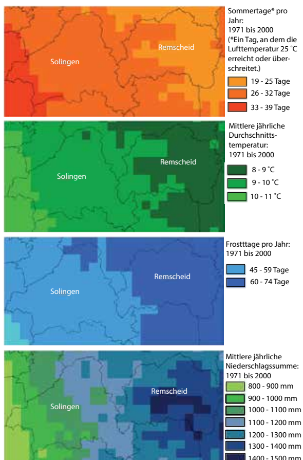
Abbildung 3: Klima-Ist-Zustand in Solingen und Remscheid (1971 bis 2000)
