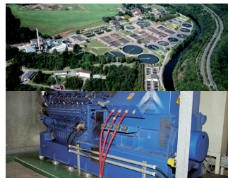
Klärgasbetriebene BHKW's (2,4 MW) des Wupperverbandes decken 70 % des Strombedarfs des Klärwerks in Wuppertal-Buchenhofen und liefern Wärme für das Klärwerk und angrenzende Liegenschaften.
